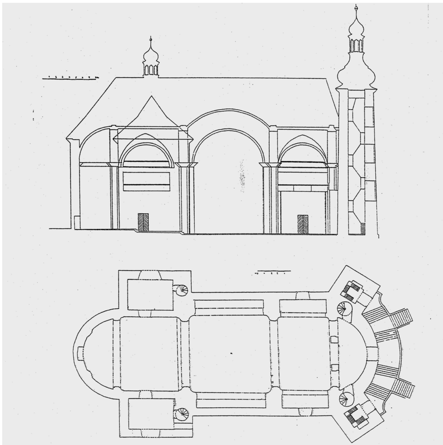
Plan et coupe longitudinale de l'église de l'Assomption à Neratov, d'après les plans de Josef Kalous de 1945 (Les archives de district d'Ústí nad Or.).
